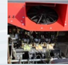
GÜÇLÜ FAN SİSTEMİ BINDING GROUP CLEANING FAN
